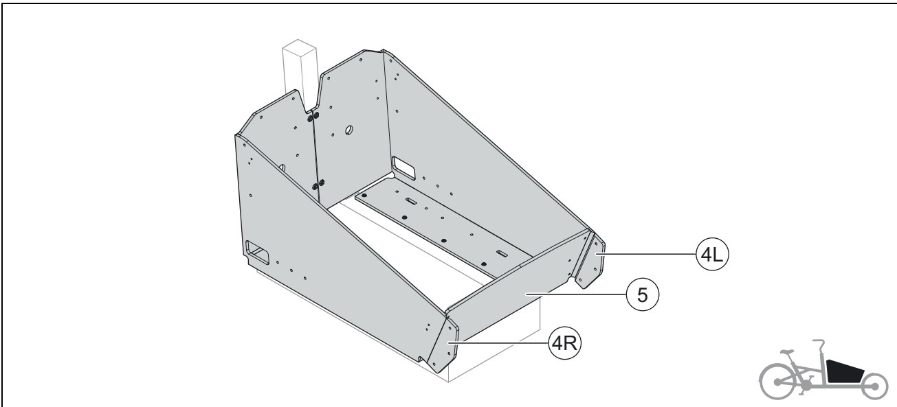
Abbildung 8: Vorderwand hochklappen
