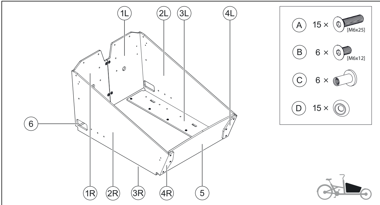
Abbildung 1: KETTLER Flexbox
