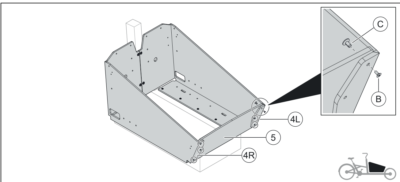
Abbildung 9: Vorderwand verschrauben
