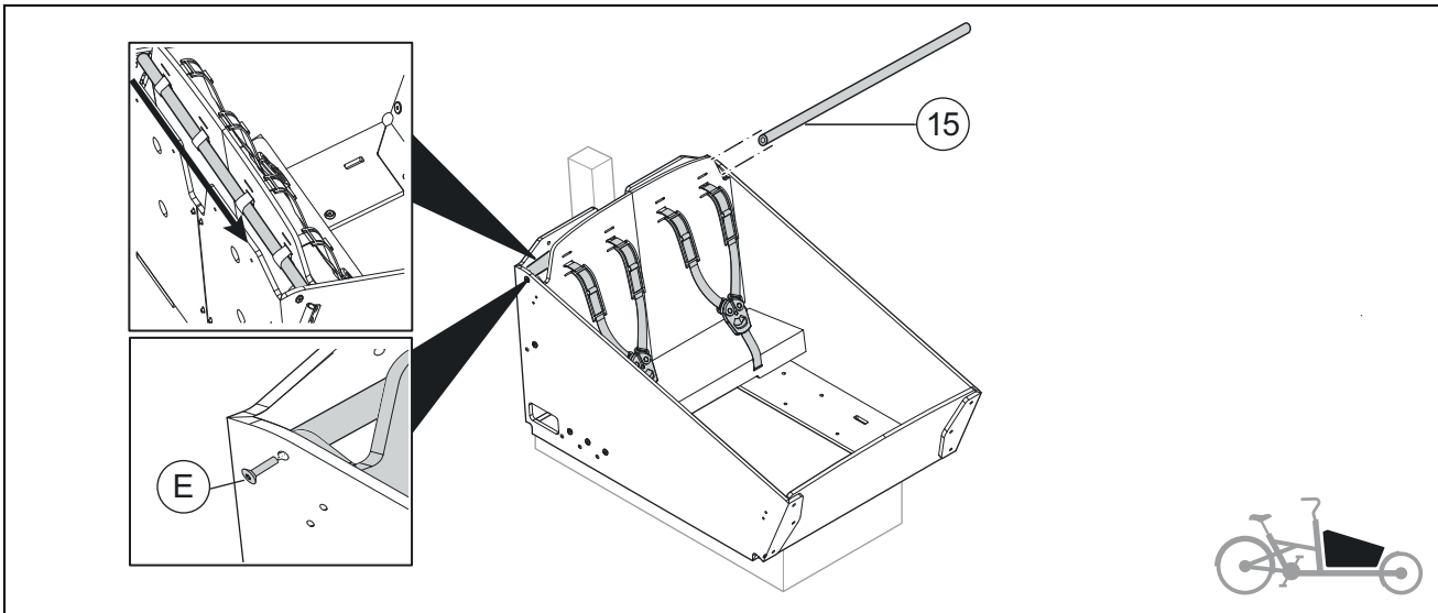
Abbildung 14: Schultergurte montieren
